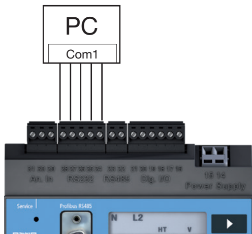
Abb. Beispiel, ein UMG604-PRO über die RS232 Schnittstelle mit einem PC verbinden.
