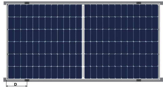
Installation eines gerahmten Moduls mit Befestigungen an den Längsseiten (Balken parallel zu den Längsseiten) (Klemmlänge \geq 40 mm)
