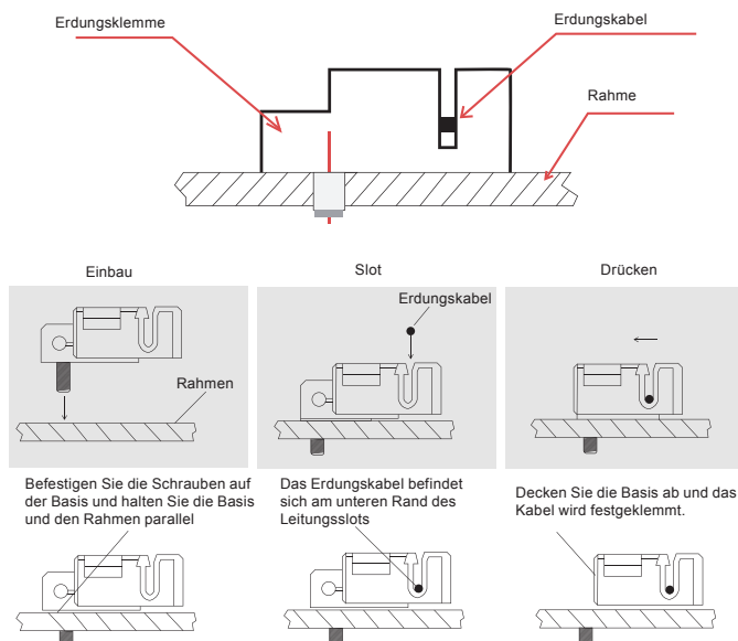
Abbildung 11 Installationsmethode der Erdungsklemme
