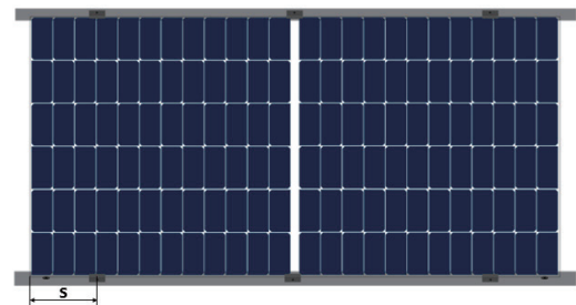
Installation eines rahmenlosen Moduls mit Befestigungen an den Längsseiten (Klemmlänge = 150 mm)
