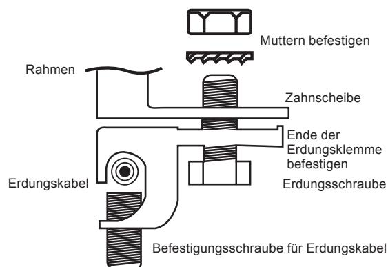
Abbildung 12 Installationsmethode der Erdungsschraube
