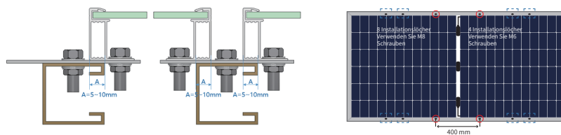
Abbildung 7 Schraubeninstallation des Bifacial-Moduls
