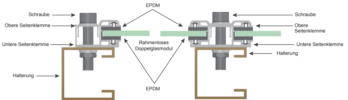
Rahmenloses Bifacial-Doppelglasmodul
