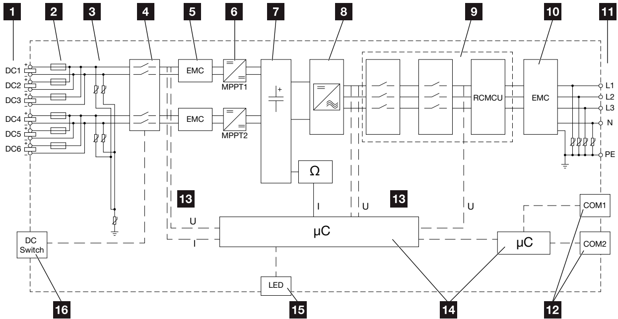
Abb. 35: Blockschaltbild PIKO CI 30
