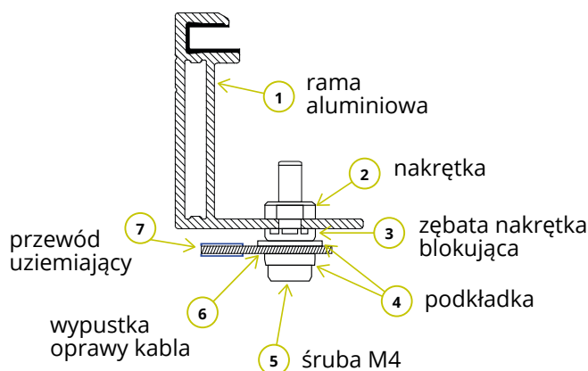
Rysunek 6 Sposób uziemienia modułu fotowoltaicznego
