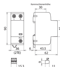
Maßbild DSH TN 255 FM
