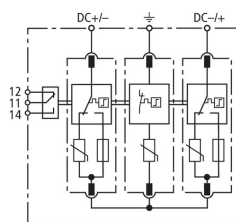
Prinzip Schaltbild DG M YPV SCI 1200 FM
