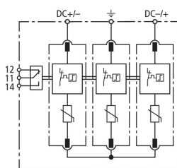
Prinzipschaltbild DG M YPV 1500 FM
