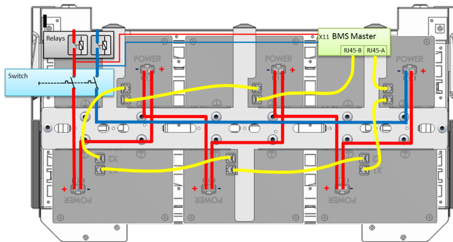
Abbildung 5: Leistungspfad mit Schalteinrichtungen und BMS
