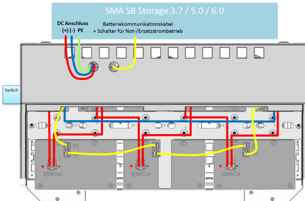
Abbildung 6: Anschluss des SMA SB Storage an AXIStorage Li SH
