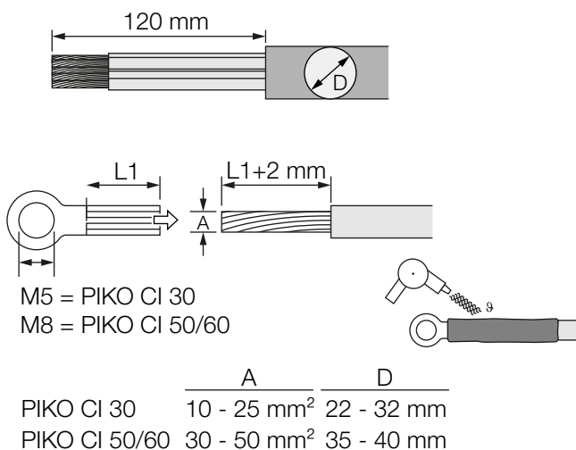
Abb. 16: AC-Leitung vorbereiten
