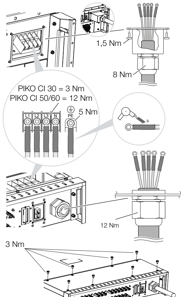
Abb. 17: AC-Anschluss abdichten
