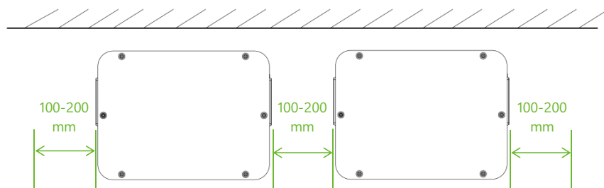
Abbildung 3-1 Mindestabstände
