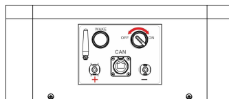
Abbildung 4-1 BDU rechte Anschlüsse
