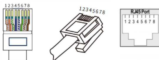
Abbildung 2-11 EXT-CAN/RS485 Stiftbelegung
