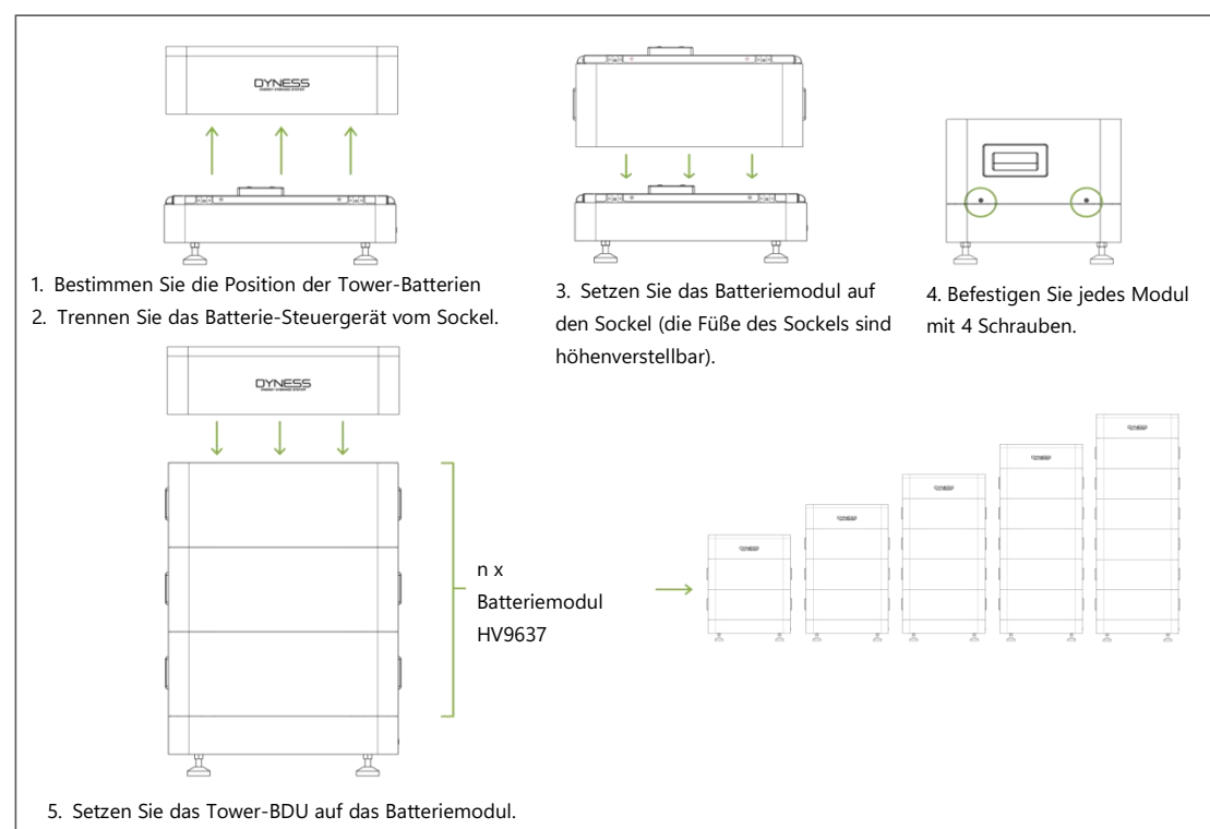
Abbildung 3-5 Mechanische installation
