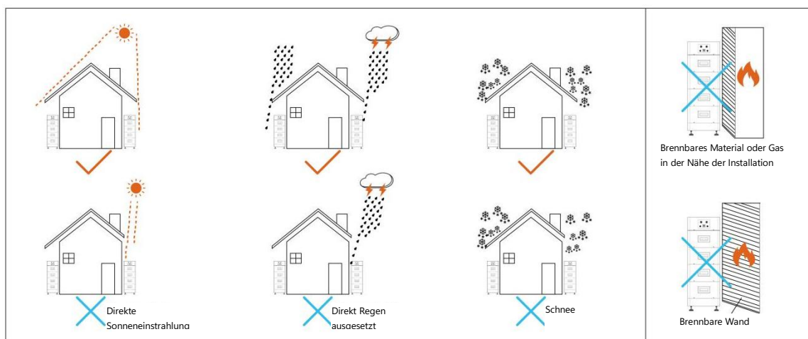
Abbildung 3-2 Installationsort
