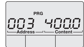
Anzeigenbeispiel 2: Die Sekundärspannung jedes Spannungswandlers an den 4 Spannungsmesseingängen beträgt 400 V.
